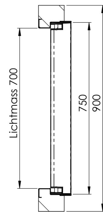
SCHNITT B-B
